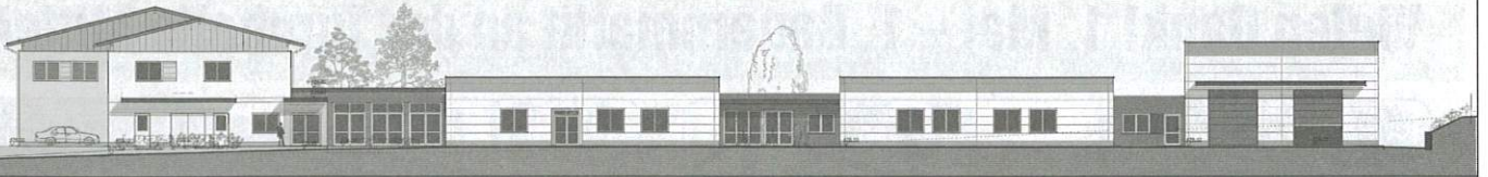
Ansicht Westseite
